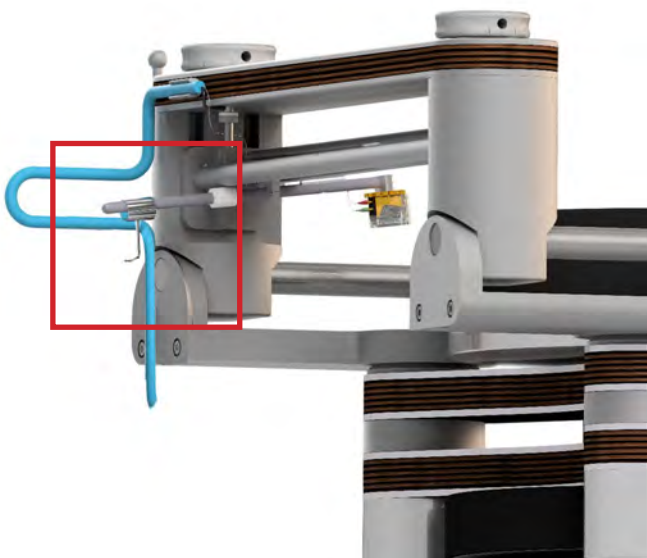
Abb. 12: Gegengewicht Einstellung
