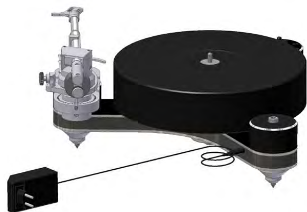
Abb. 11: Verbindung Netzteil und Motor
